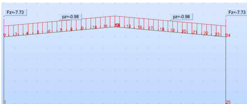
Fig. 2 Dead load
