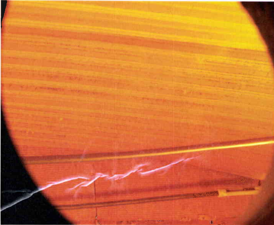
Bild 7: Zustand des Probekörpers an der beflammten Unterseite in der 15. Versuchsminute
