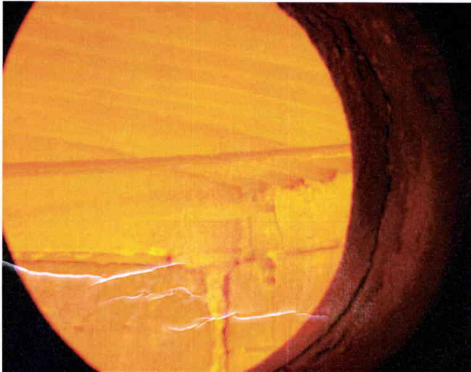
Bild 11: Zustand des Probekörpers an der beflammten Unterseite in der 90. Versuchsminute
