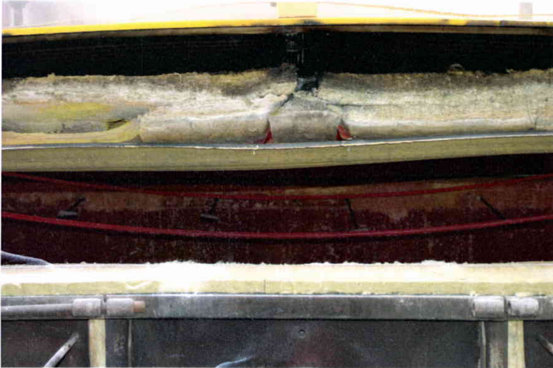
Bild 13: Ansicht Dachaufbau nach Versuchsende und Wegnahme der Belastung im mittleren Bereich
